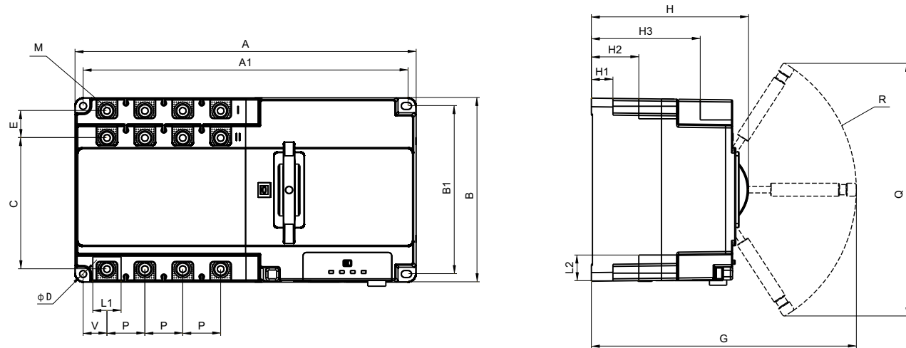
XLDS2T-250/630外形图
