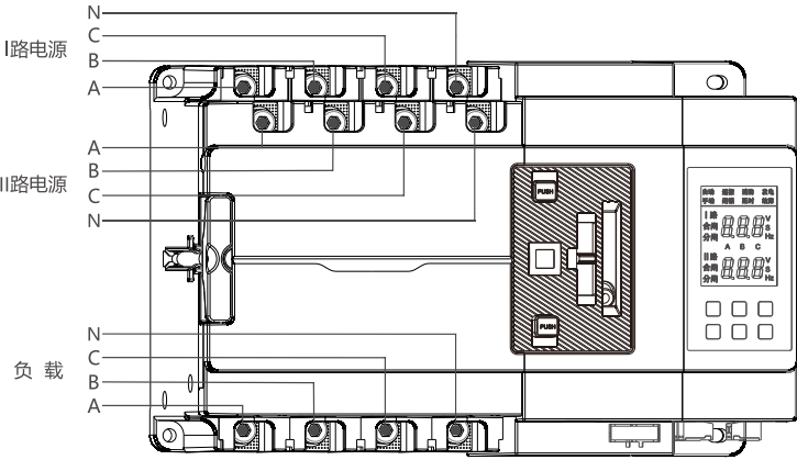
图6-2 4P产品相序定义图
