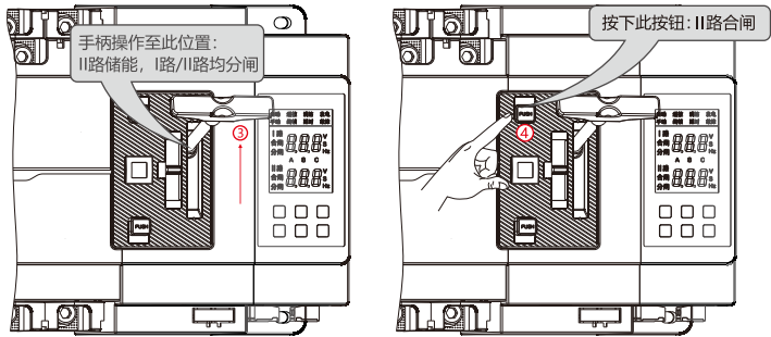
图4-3 三段式开关操作图
