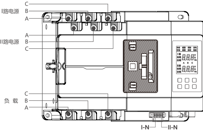
图6-1 3P产品相序定义图
