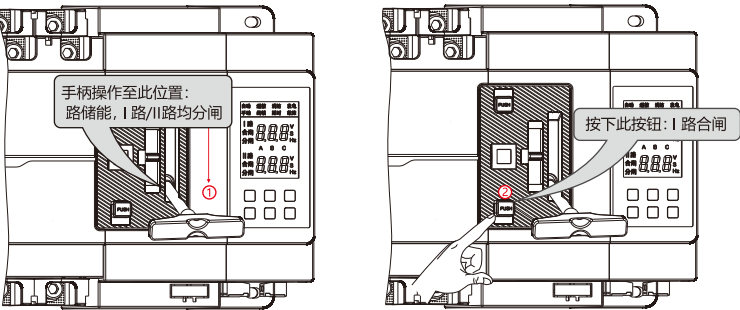
图4-2 三段式开关操作图
