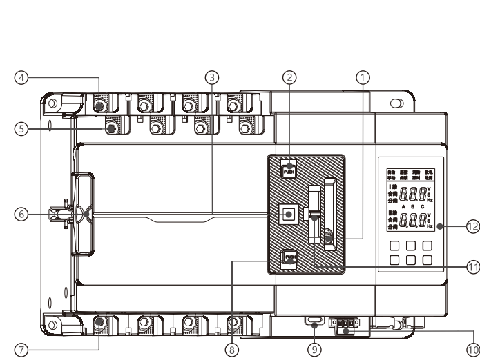
图1-1 整体式外形图
