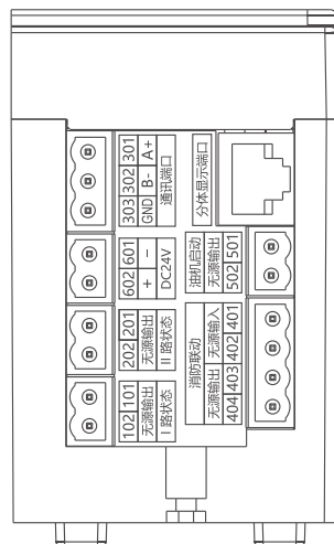
图5-2 B型控制器
