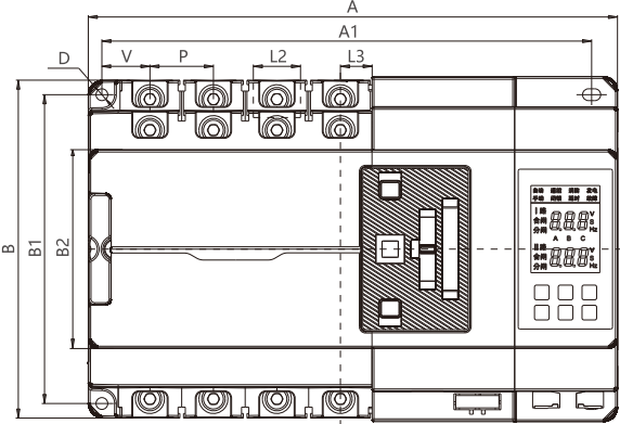
图3-1 整体式主视图
