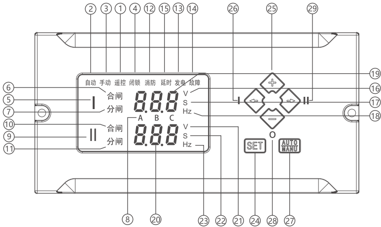
图2-2 分体式控制器
