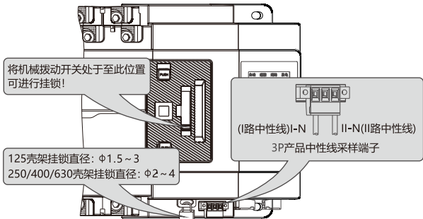
图4-4 挂锁及3P产品中性端子接线图
