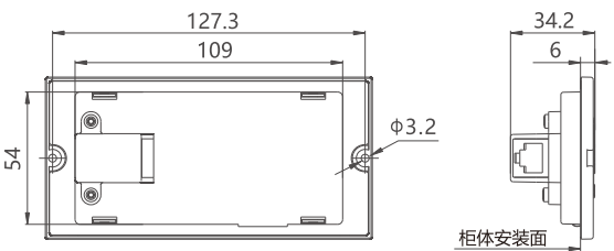
图3-4 分体式液晶屏控制模块尺寸
