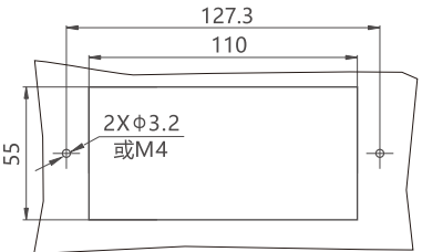
图3-5 分体式液晶屏控制模块柜体开孔尺寸
