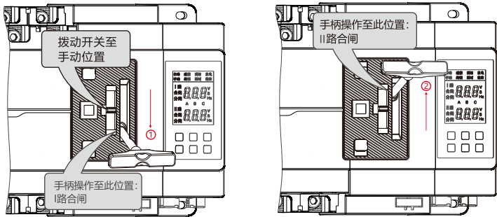
图4-1 两段式开关操作图
