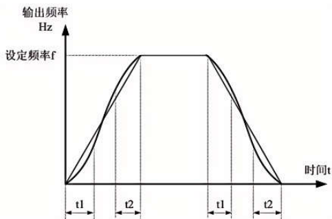
图 F01-1 曲线加减速 A 示意图
