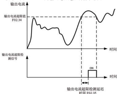
图 F01-11 输出电流超限检测示意图
