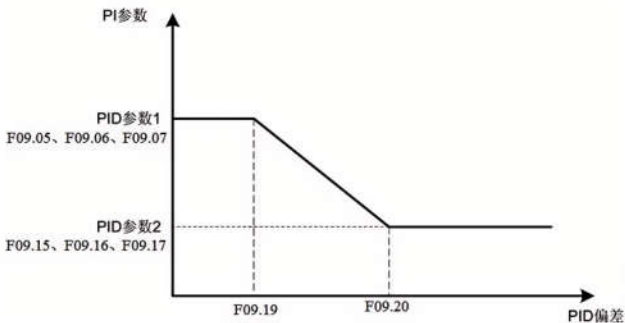
图 F09-1 PID 参数切换
