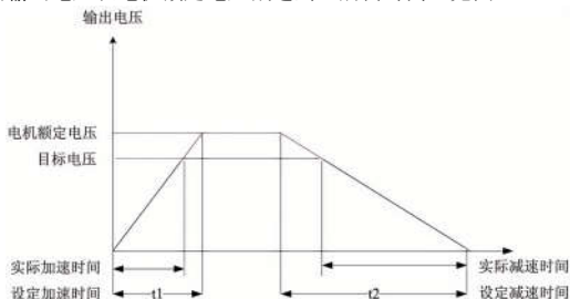
图 F06-3 V/F 分离示意图
