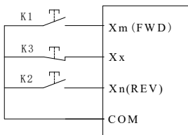
图 F07-4 三线式控制模式 1 示意图
