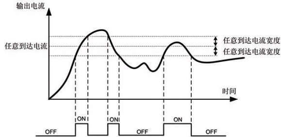
图 F01-12 任意到达频率检测示意图
