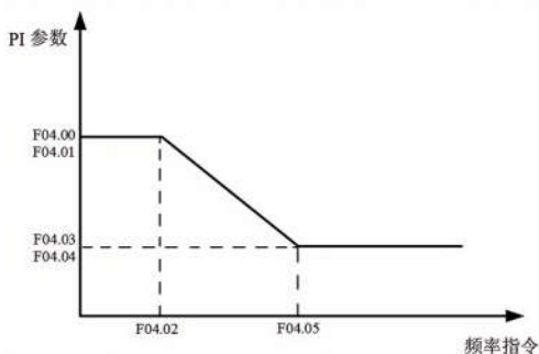
图 F04-1 PI 参数示意图
