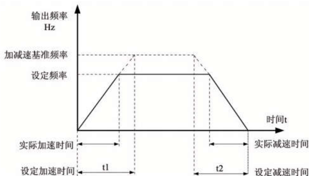
图 F00-1 加速时间和减速度示意图
