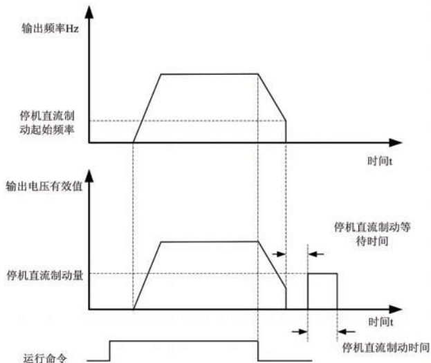
图 F01-3 停机直流制动示意
