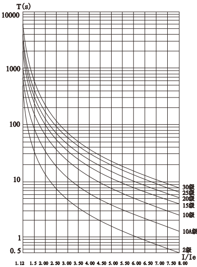
IEC60974-4-2电机热态保护曲线
