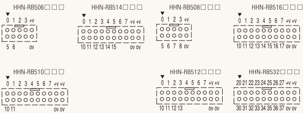
配线图 Wiring Diagram
