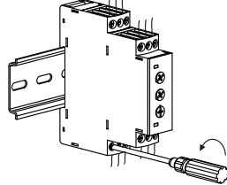
(5) 拧松接线螺钉并拆除导线
