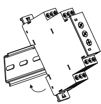
(2) 将产品扣入导轨
