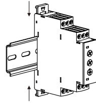
(3) 合上导轨卡
