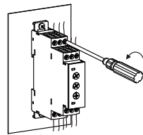
(9) 拧松接线螺钉并拆除导线
