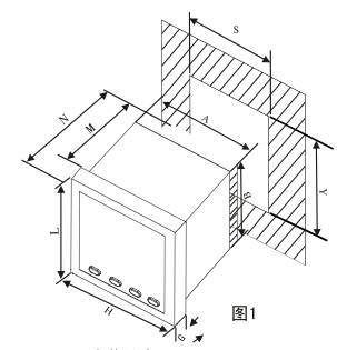
安装尺寸: A×B 开孔尺寸: S×Y 面板尺寸: L×H (单位:mm)
