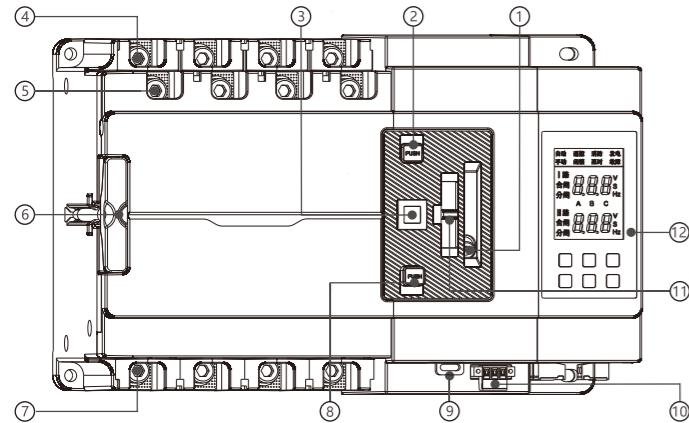
图1-1 整体式外形图
