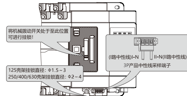
图4-4 挂锁及3P产品中性端子接线图
