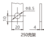
图3-3 产品接线铜排尺寸
