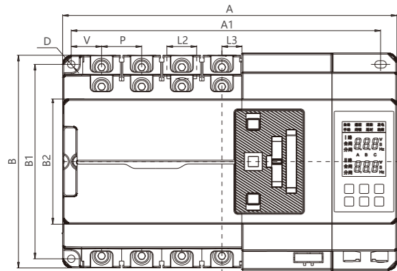
图3-1 整体式主视图
