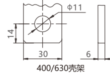
400/630壳架
