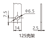
125壳架
