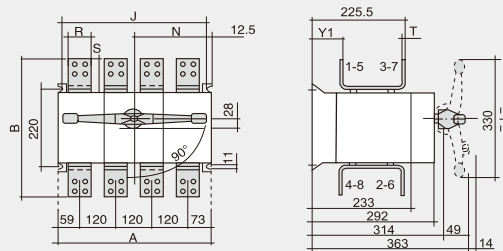
XLGL-2000~2500A正面直接操作 Direct operation on front face XLGL-2000~2500A
