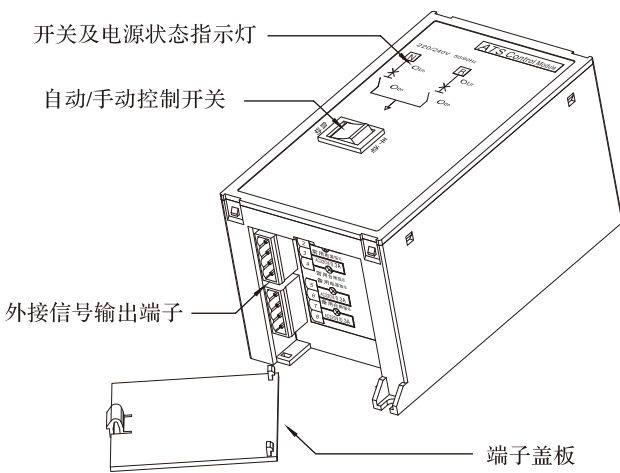
控制器结构
