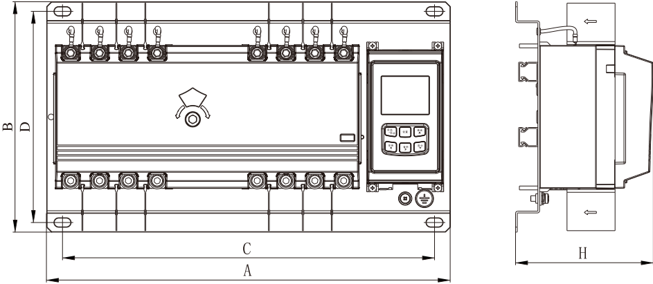
XLDQ3NM 外形图
